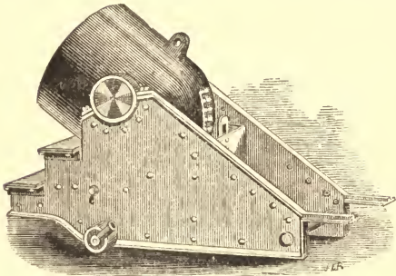
FIG. 7.—13-inch Mortar.
